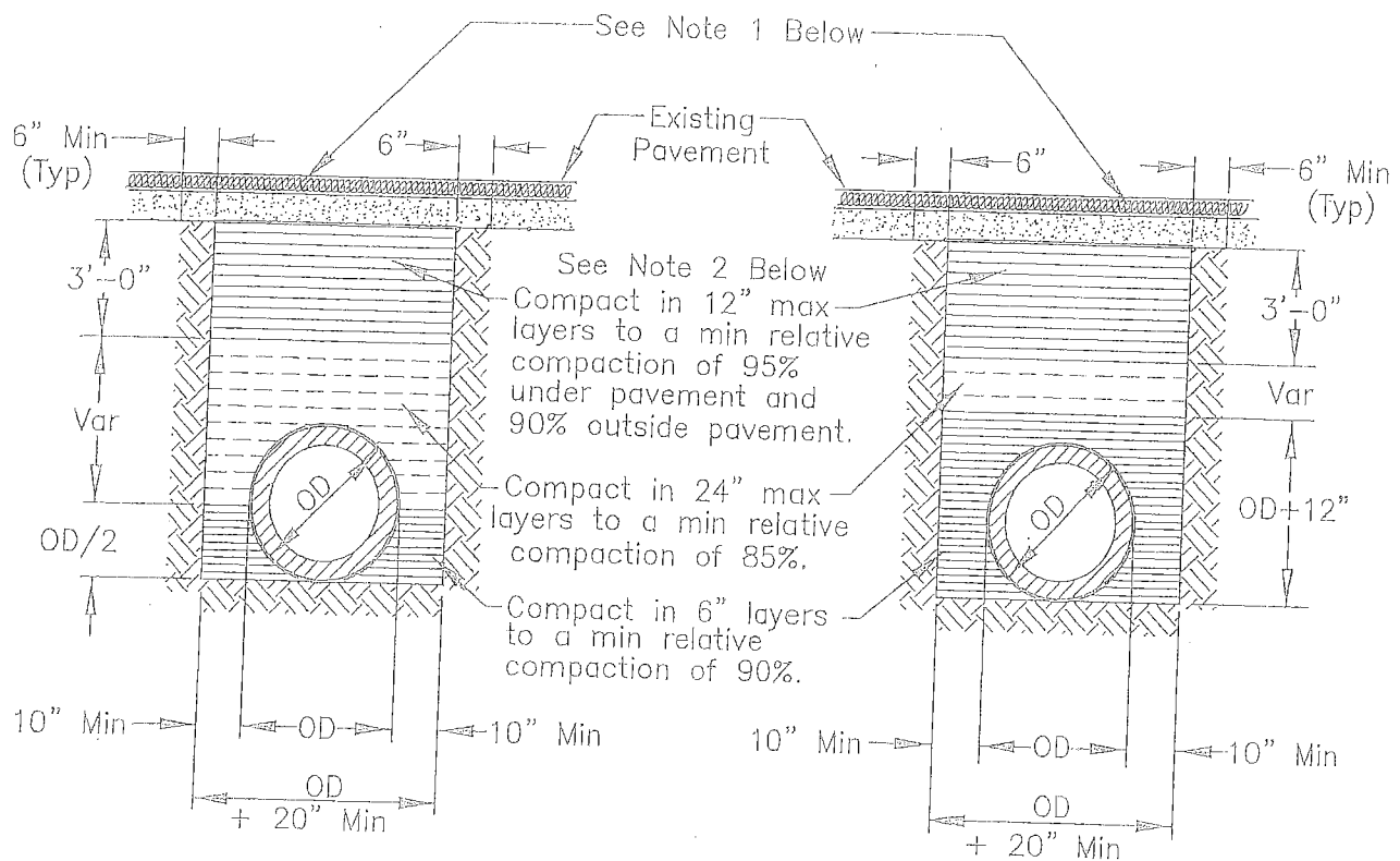
RIGID CONDUIT
